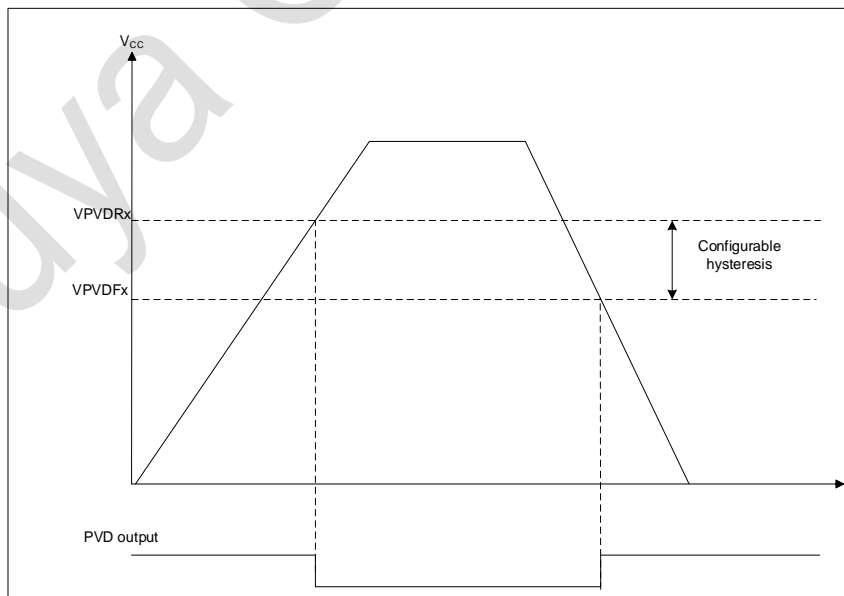
图 2-4 PVD 阈值
