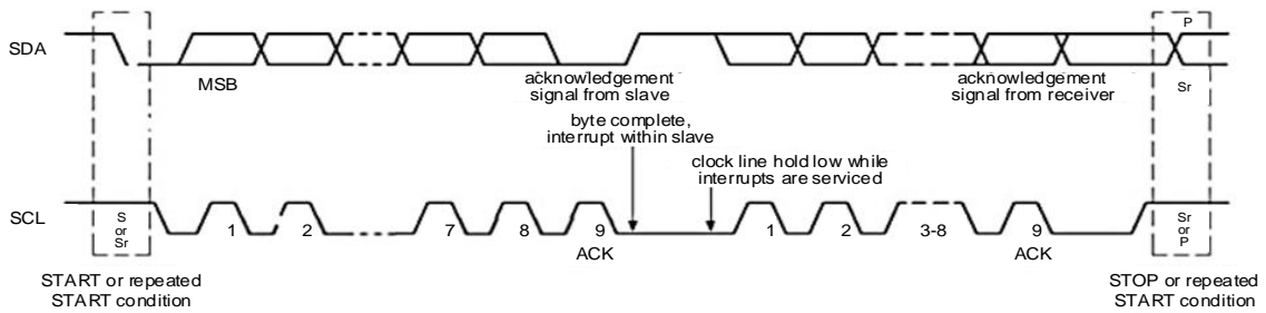
图 5-9 I 2 C 总线的响应
