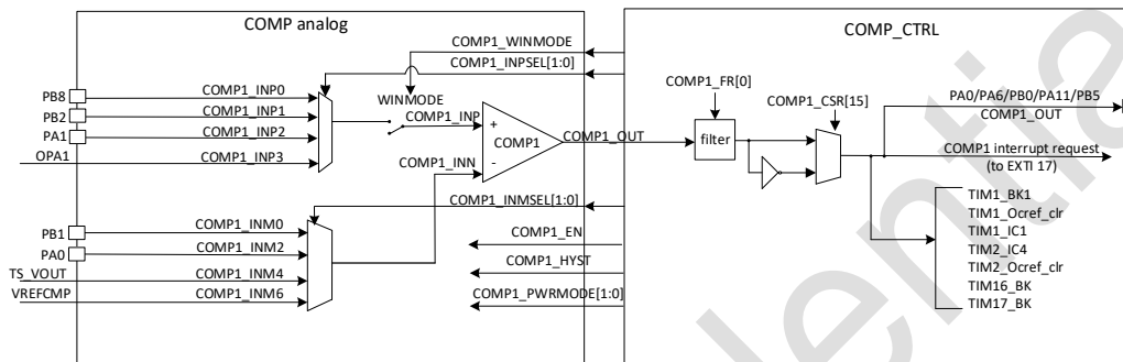
图 2-5 COMP 框图
