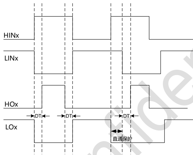
图 5-5 直通保护
