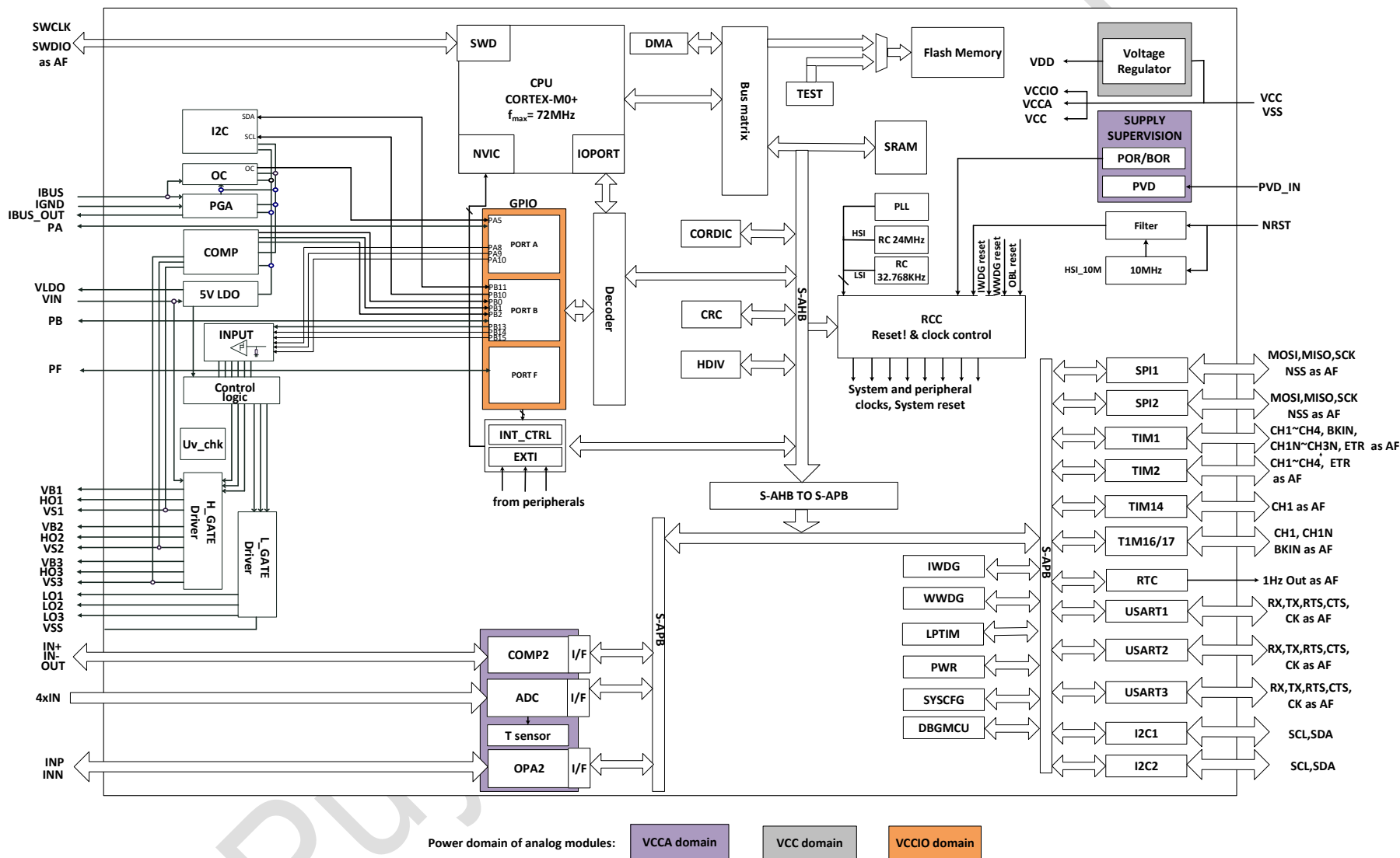
图 1-1 功能模块
