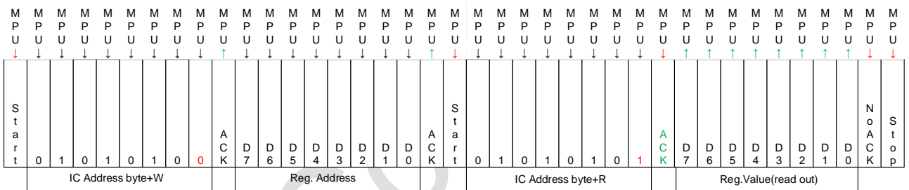
图 5-12 读命令格式
