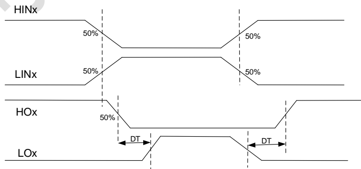
图 5-6 死区功能
